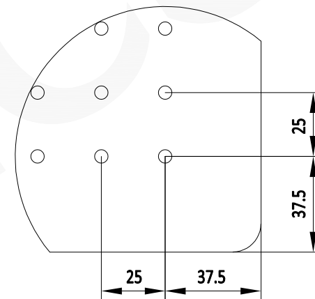
局部视图A 比例1:2
