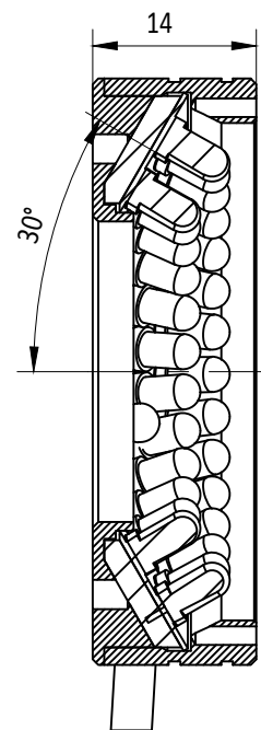
剖视图 A-A
