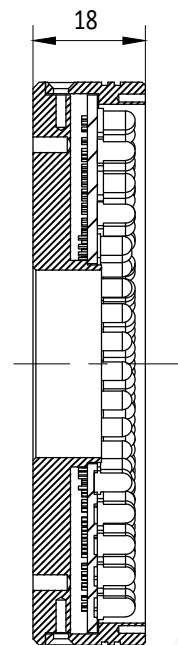
剖视图 A-A
