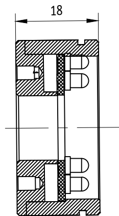
剖视图 B-B
