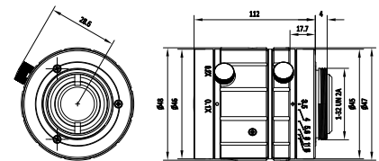
尺寸图
