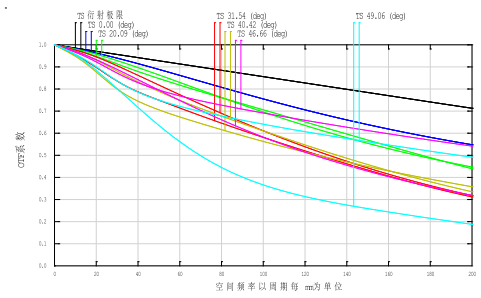
相对照度
