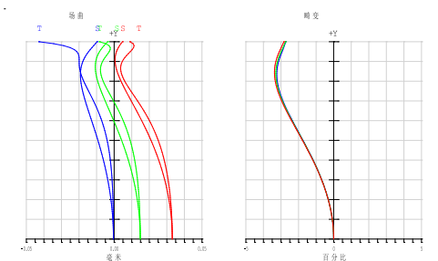
畸变率
