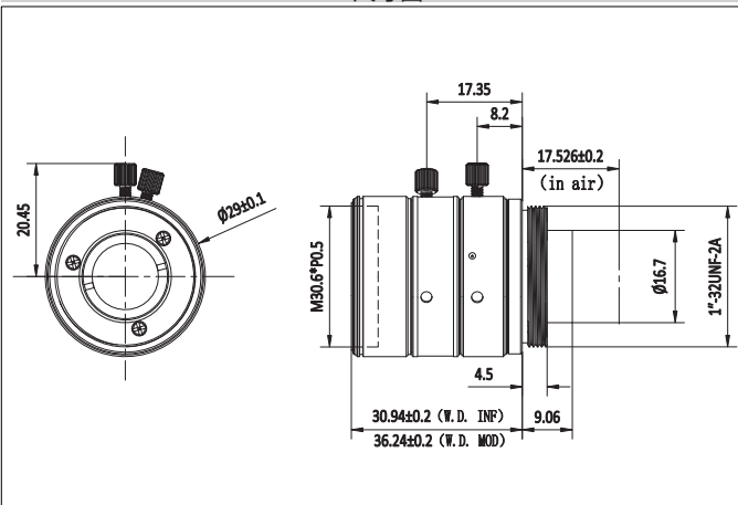
尺寸图
